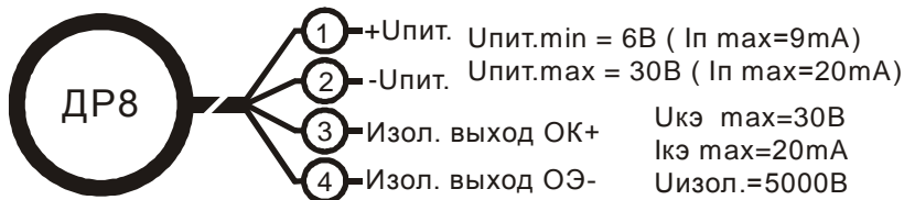
Рис.2 Обозначение выводов датчика ДР8М
